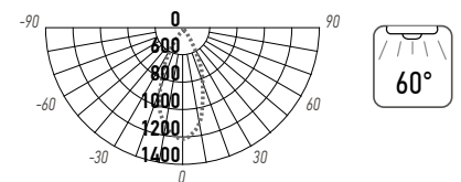
MTR16 1412 12W
