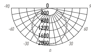
PWP-C3 SPEC
