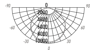
PSL 08 100W 120°
