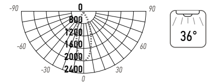
MTR16 1212 12W
