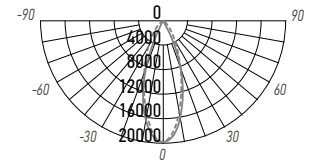
PTR 0530 30W
