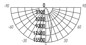
PTR 1732 32W
