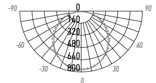
PWP-OS 36W
