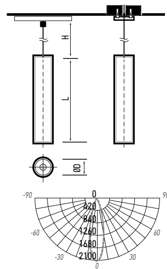
PTR 2310W
