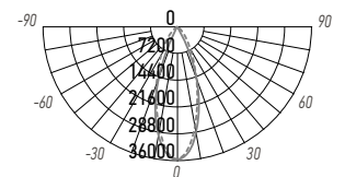
PTR 0620 20W
