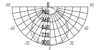
PTR 1935 35W
