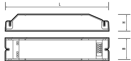
РЕРР40-1.0Н U IP20 (Габаритные размеры)
