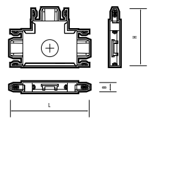
MTR16 CT-BL Коннектор черный T-обр.
