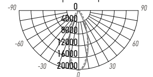
PTR 1335 35W
