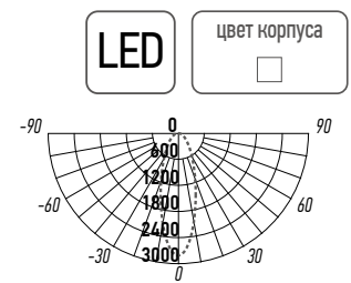
PSP-S 412 2X8W
