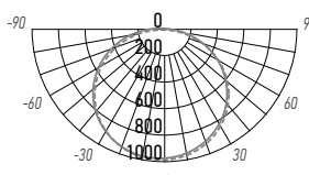
РРО-04 1200 36W
