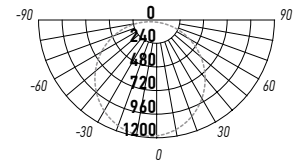
PSO-01 36W
