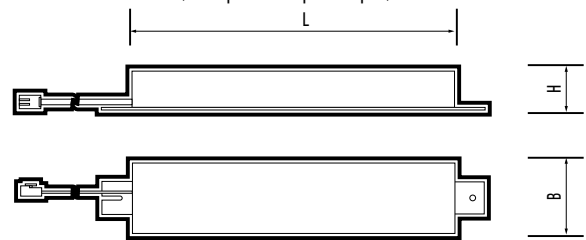
РЕРР40-1.0Н U IP20 (Габаритные размеры аккумулятора)
