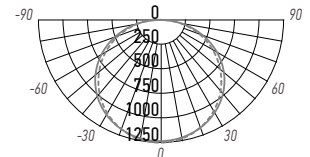
РВН-РС2 12W
