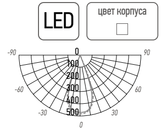
PSP-R 7W
