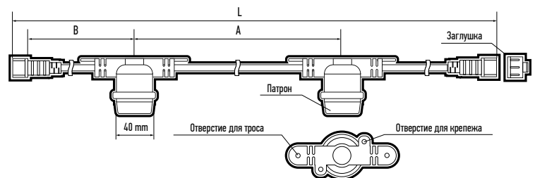
Гирлянда PBL
